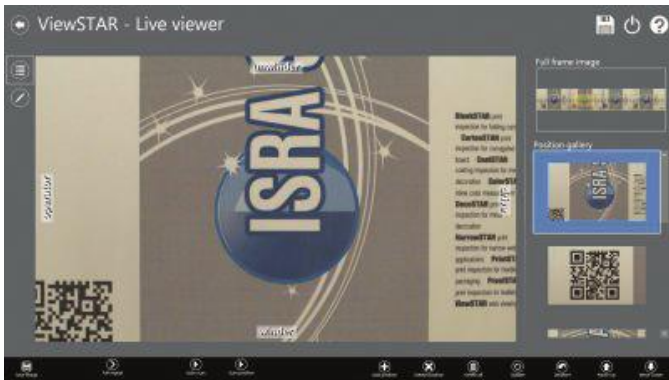
651_2 ViewSTAR bietet eine realitätsgetreue Wiedergabe des tatsächlichen Druckbilds auch bei hohen Bandgeschwindigkeiten
